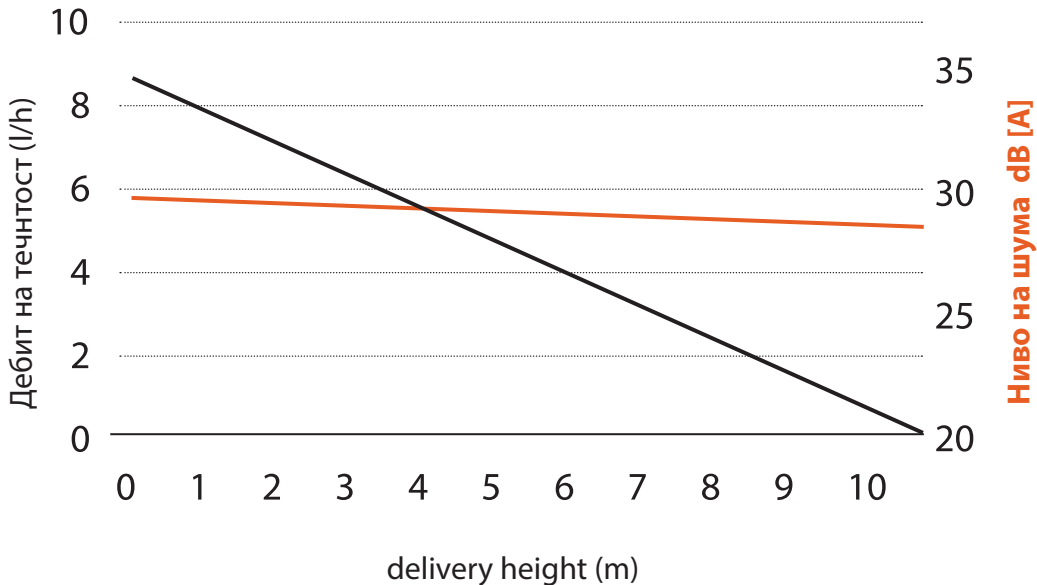
Диаграма на мощността и звуковото налягане
