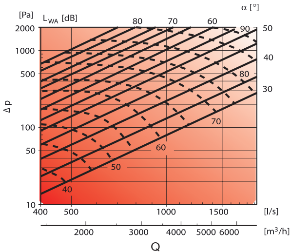
AKH Ø500
