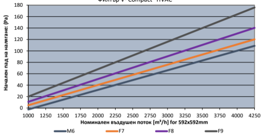
Филтър V- Compact "HVAC"
