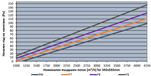
Филтър V- Compact "ENERGY"
