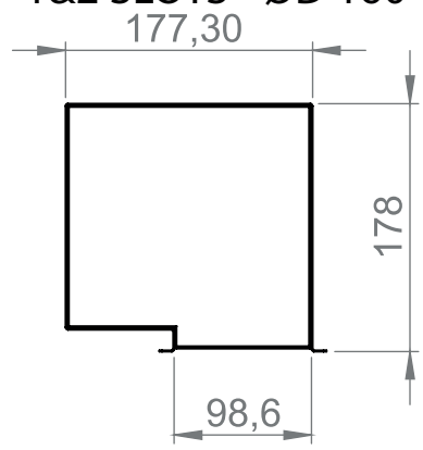
1&2 SLOTS - ØD 160
