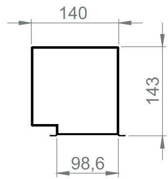
1&2 SLOTS - ØD 125
