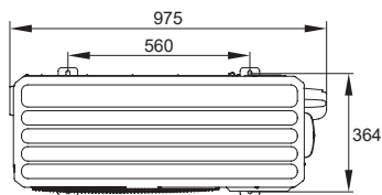
■ GRS-CQ6.0Pd/NhH2-E(O)
