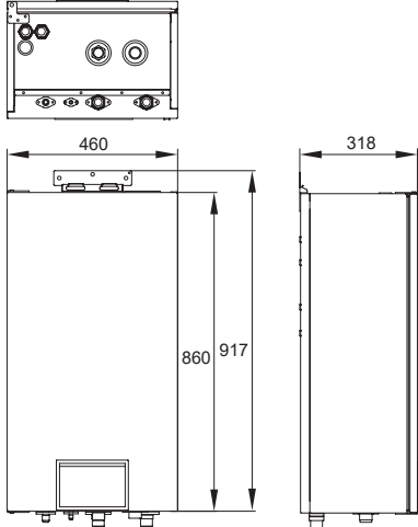
■ GRS-CQ6.0Pd/NhH2-E(I) - GRS-CQ16Pd/NhH-E(I)/GRS-CQ16Pd/NhH-M(I)
