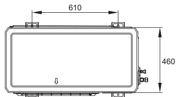
■ GRS-CQ16Pd/NhH-E(O)/GRS-CQ16Pd/NhH-M(O)
