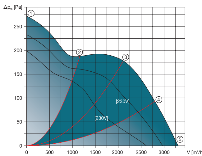
EM 400 E4M 01
