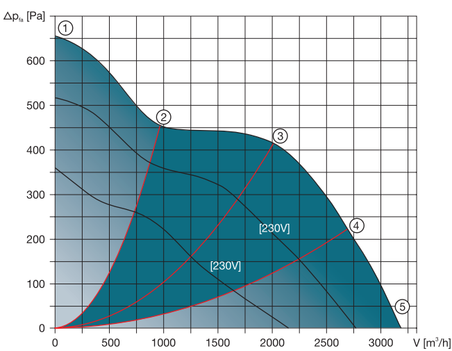
EM 315 E2M 01
