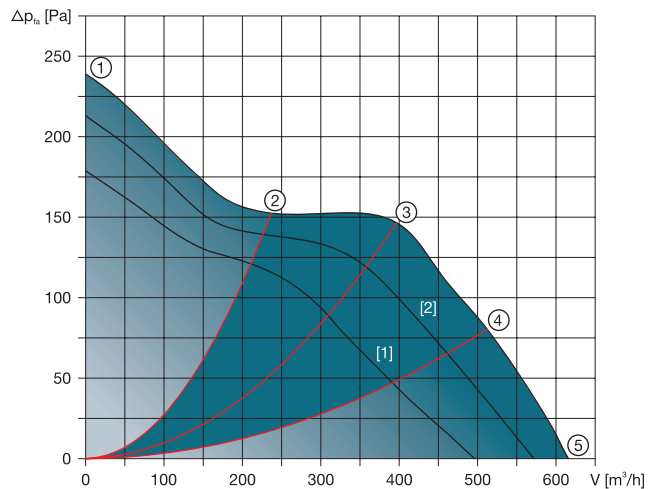
EM 160 E2M 01
