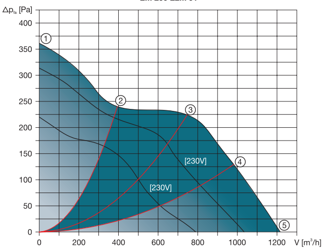
EM 200 E2M 01
