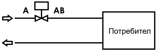
Вентил с променлив поток
