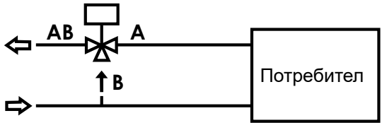
Смесителен вентил в режим на пренасочване
