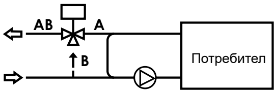
Смесителен вентил за постоянен поток
