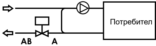
Вентил с постоянен поток
