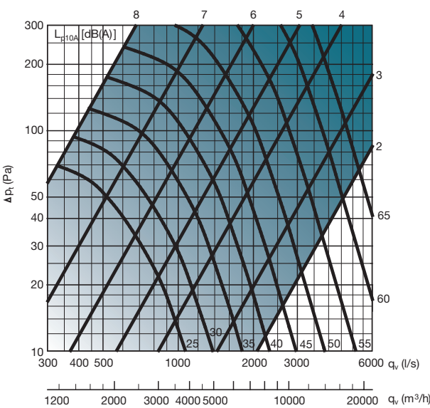
IRIS 630
