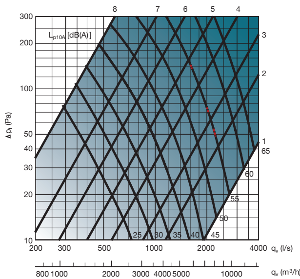
IRIS 500
