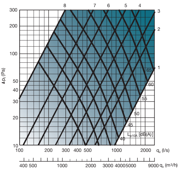
IRIS 400
