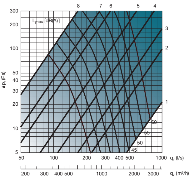
IRIS 250
