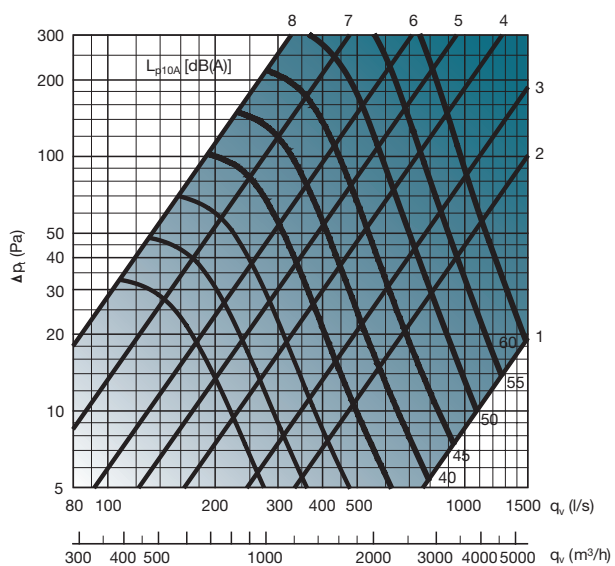
IRIS 315
