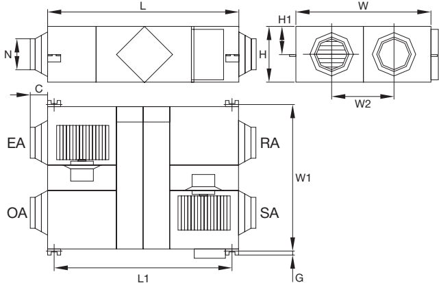
■ CHRU-TF 150(C) - CHRU-TF 650(C)
