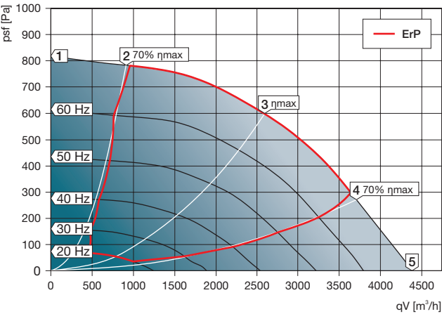
KCF-N 355 D4 40
