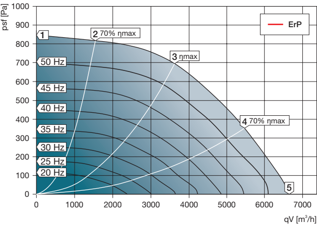
KCF-N 450 D4 40
