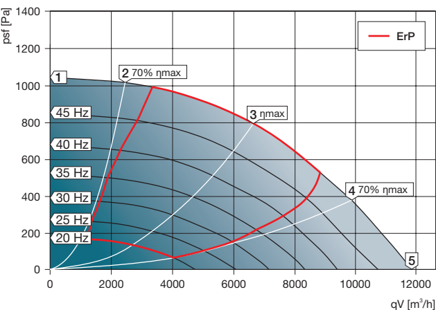
KCF-N 560 D4 40
