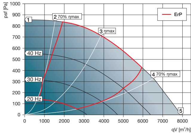
KCF-N 500 D4 40
