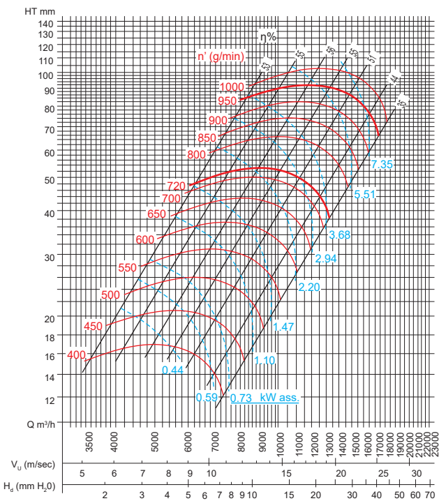
VSB 60 (55/145)
