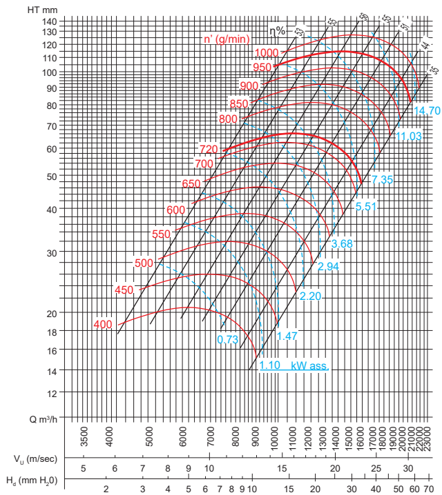
VSB 60 (60/160)
