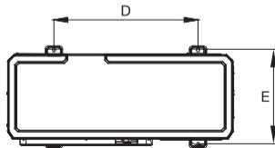
■ GMV120WL/C-T - GMV160WL/C-T
