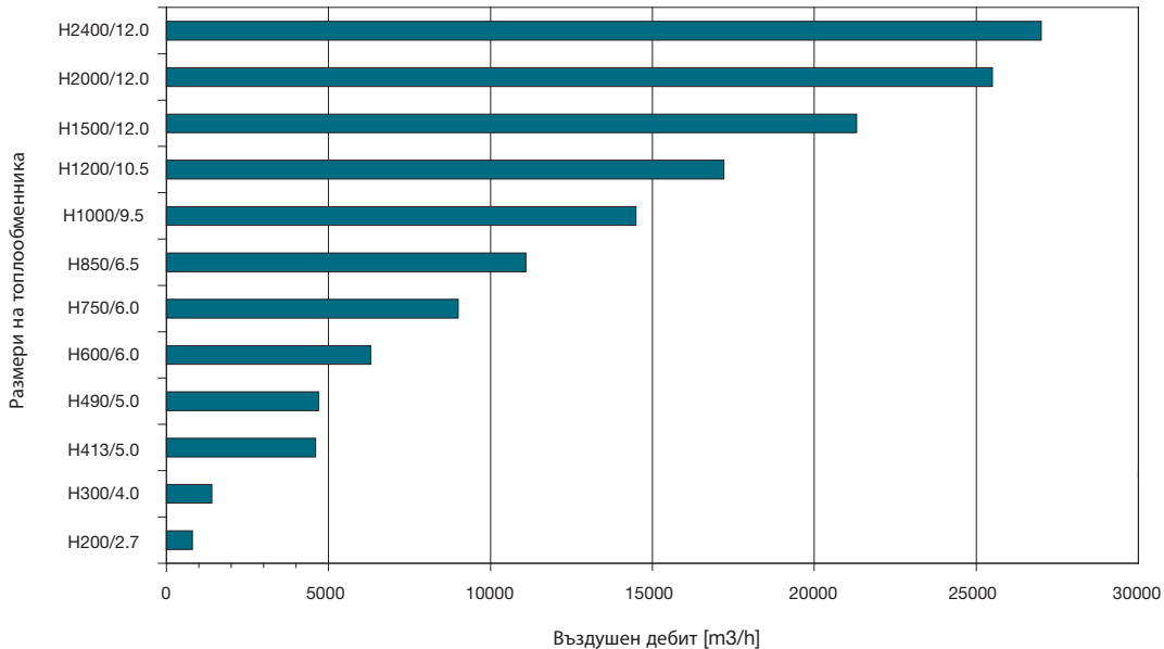
Диаграмата показва приблизително максималния въздушен дебит при съпротивление 250 Pa, при B = 1000 mm, за различните размери на топлообменника
