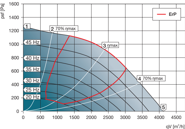
KBF-N 315 D2 T40
