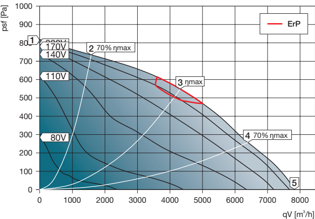
KBF-N 500 E4 T21
