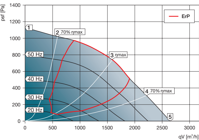
KBF-N 250 D2 T40
