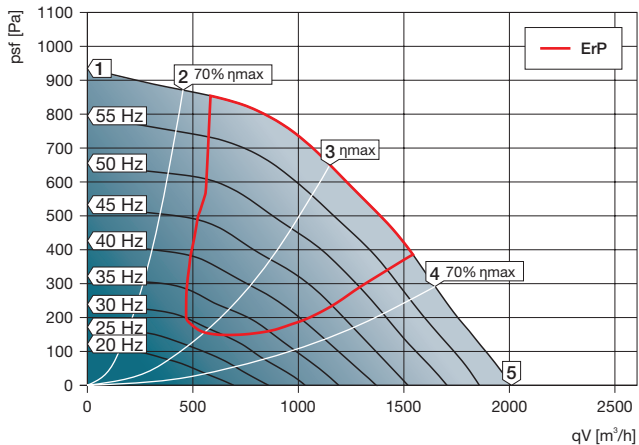
KBF-N 225 D2 T40
