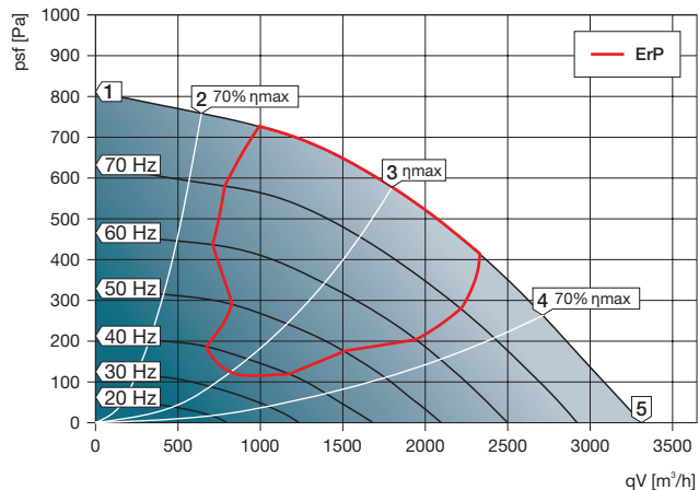
KBF-N 315 D4 T40
