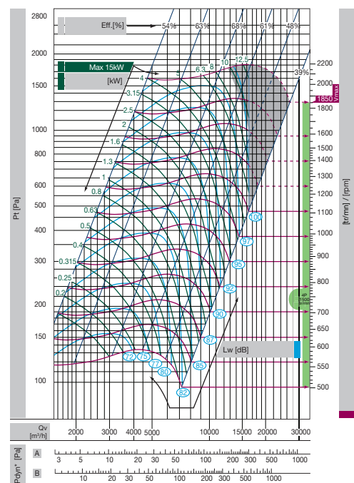
CFV 355 A
