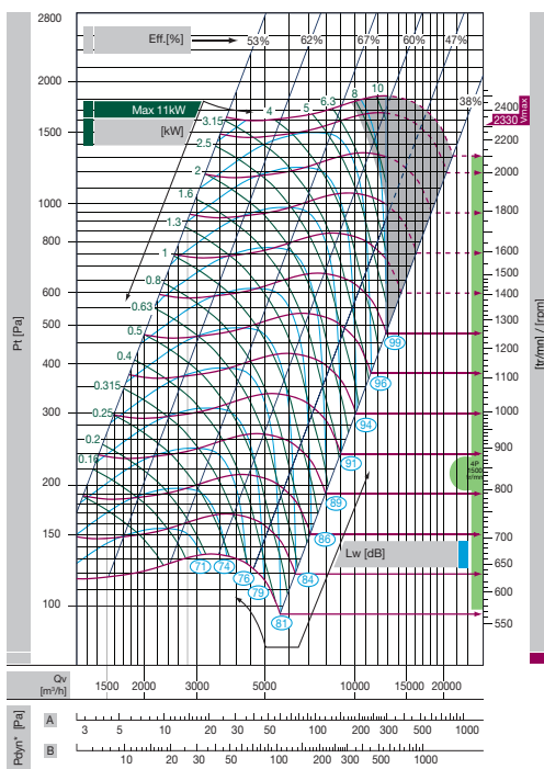
CFV 315 A
