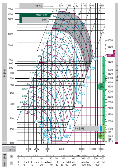
CFV 315 R
