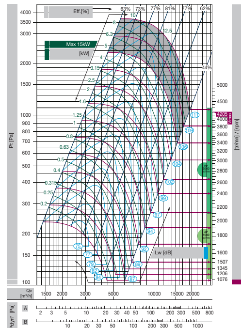
CFV 355 R
