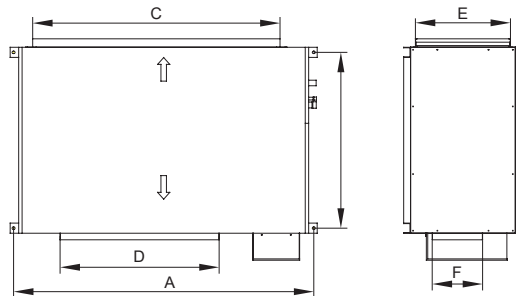
■ GMV-NX450P/A(X4.0)-M
